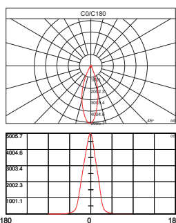
CURVA FOTOMETRICA
